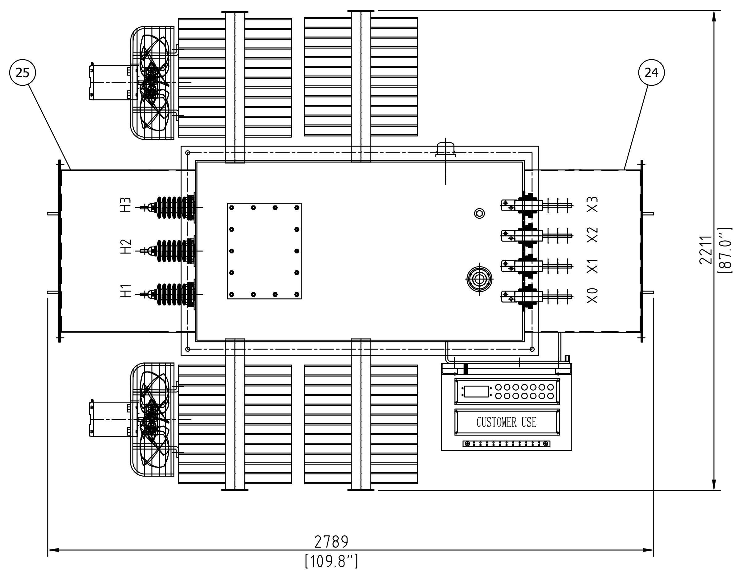
H.V terminal
